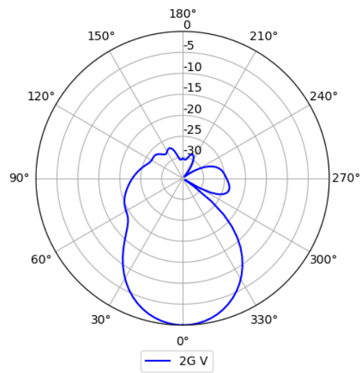
2.4GHz (Vertical)
