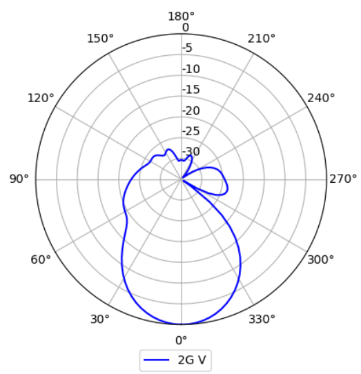
5GHz (Vertical)
